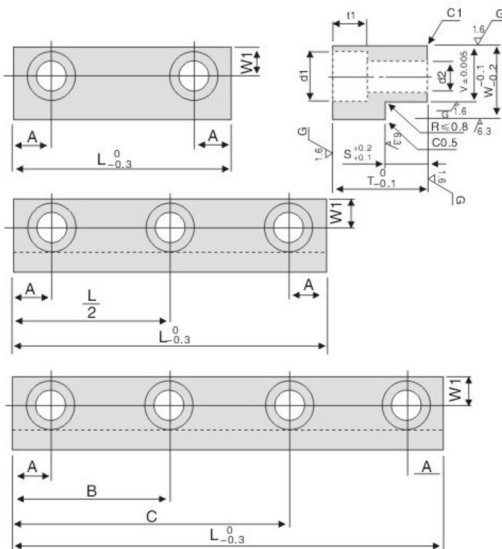
■ 螺栓孔尺寸表 bolt hole's size
